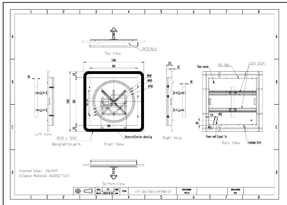
Figur 1: Sammenstillingstegning (GA)
