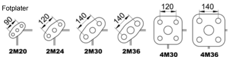
Prefabrikkerte fundamenter
