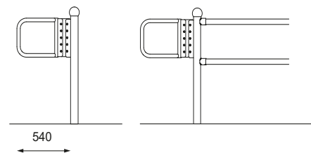
Rekkverksender for perronger
