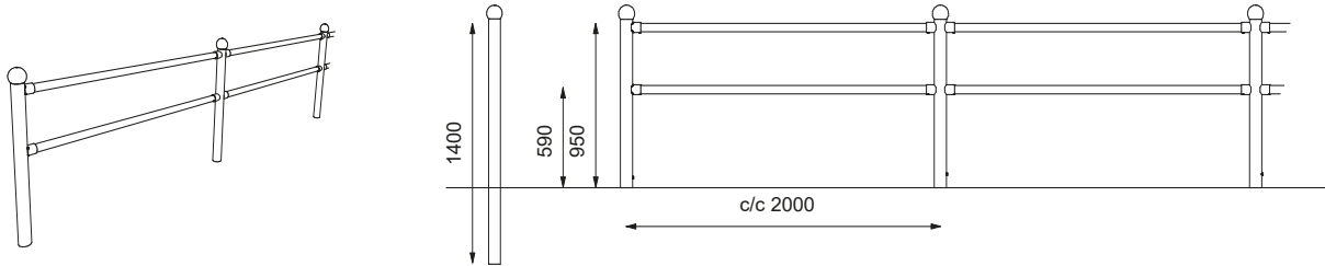
ADAPTER stolpeende med kule
