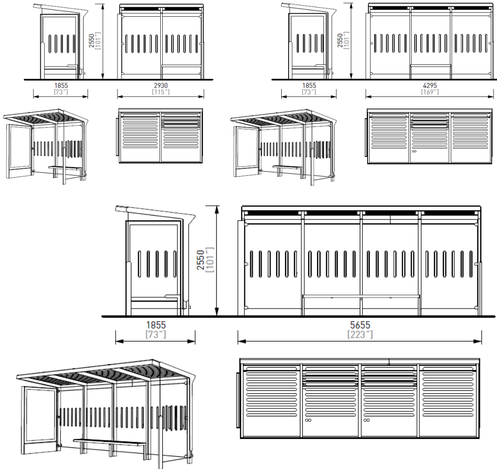
Mulighet for USB-ladepunkt ved setet. 75095000185 AE Aureo USB for leskur
