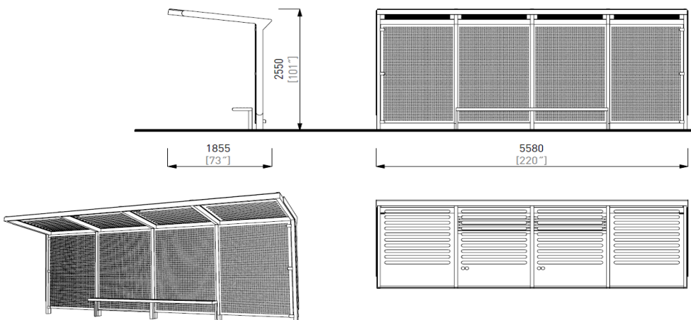
Bildet viser AE400-SP m sidevegg og Citylight
