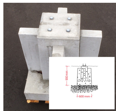
Prefabrikeret fundament
