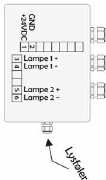
Kobling i koblingsboks
