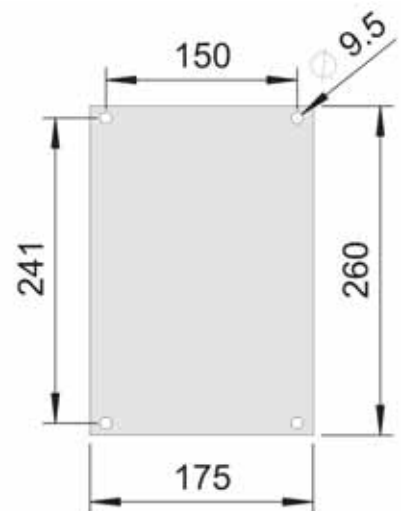
Koplingsboks brakett monteres på veggen.
