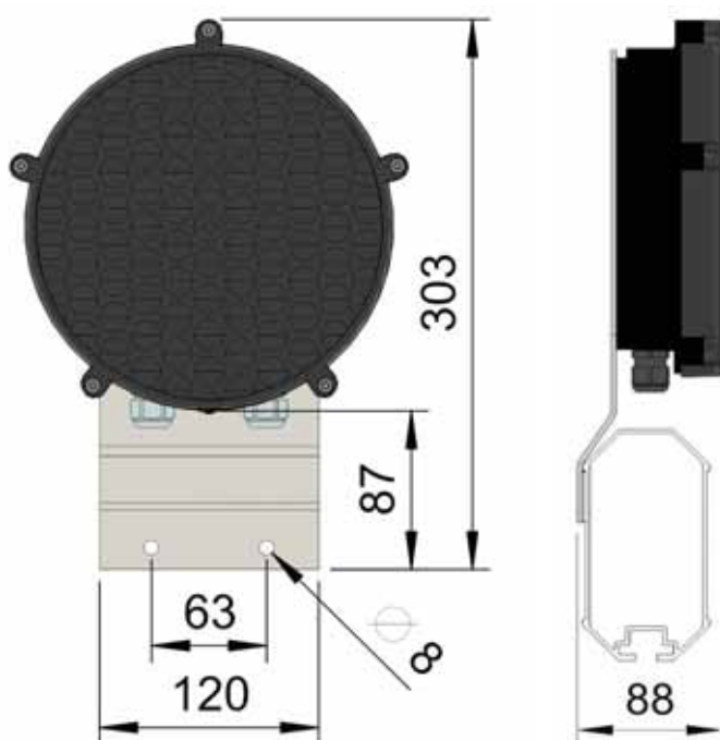
Feste for montering på bom
