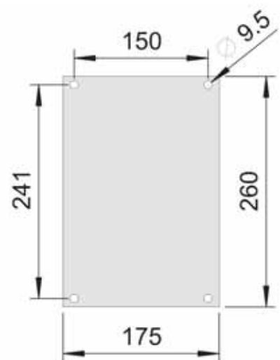
Koplingsboks brakett monteres på vegg.
