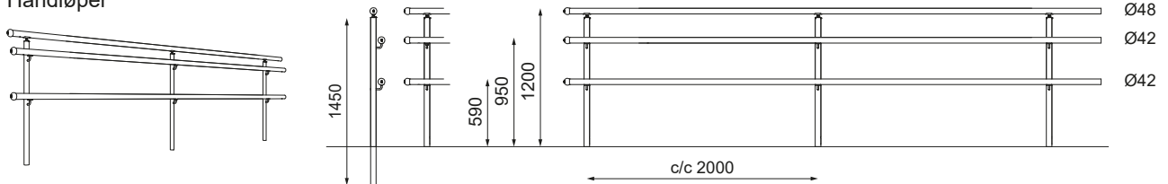
Håndløper
