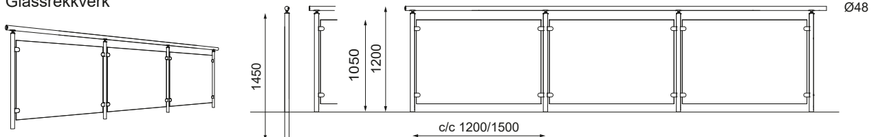
Glassrekkverk
