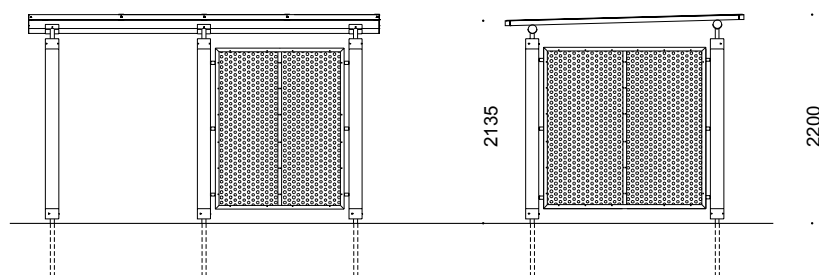
R 1000 med plan tagkonstruktion
