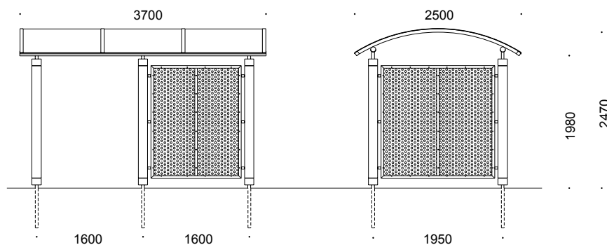
R 1000 med buet tagkonstruktion
