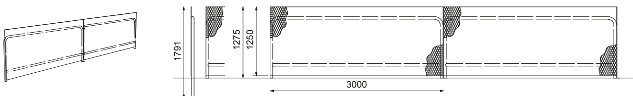
Nett med vertikale masker: Mellomstore masker (M) = 62x28 mm
