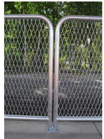
Nett med vertikale masker: Små masker (S) = 32x12 mm
